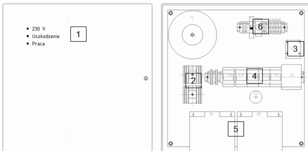
Rys. 1. Moduł rozszerzający (po lewej - widok na drzwiczki, po prawej wewnątrz obudowy wersja mcr R0448-4).
